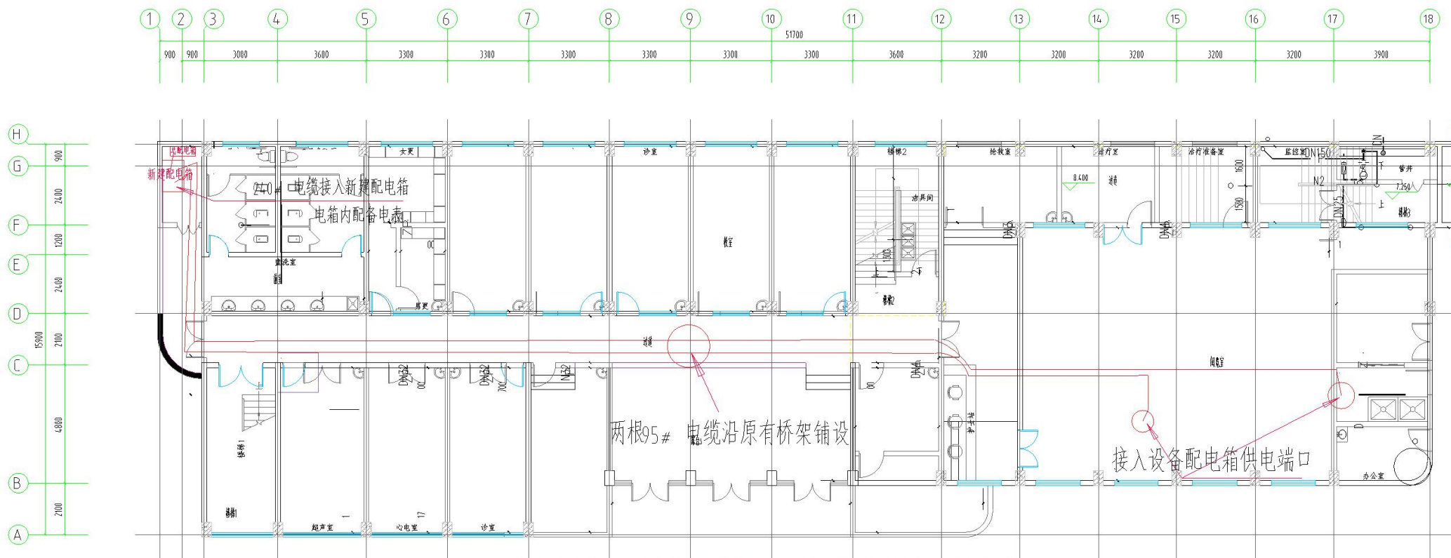
广元市第一人民医院老院区一号楼加装供电电缆项目 电缆线路走向示意图
